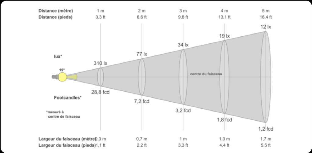
Angle 19° à 30cm Ø 10cm – 3440 lux / à 50cm Ø 17cm – 1239 lux - 3000K
